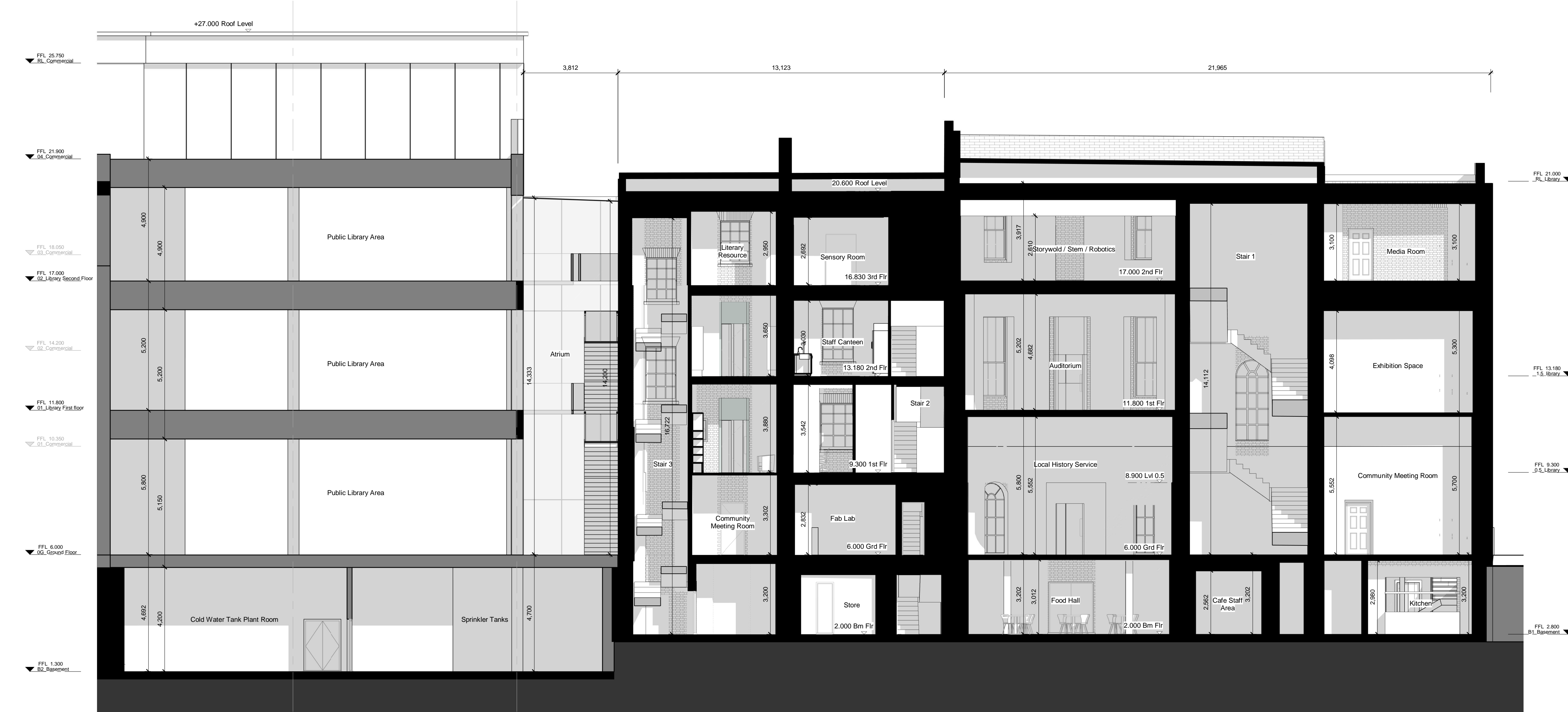
2 Section B-B SCALE: 1 : 100
