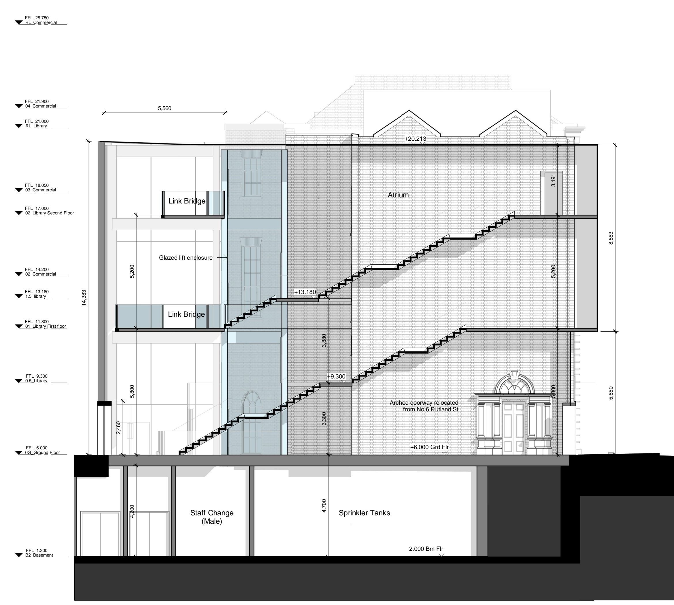
1 Section A-A SCALE: 1 : 100
